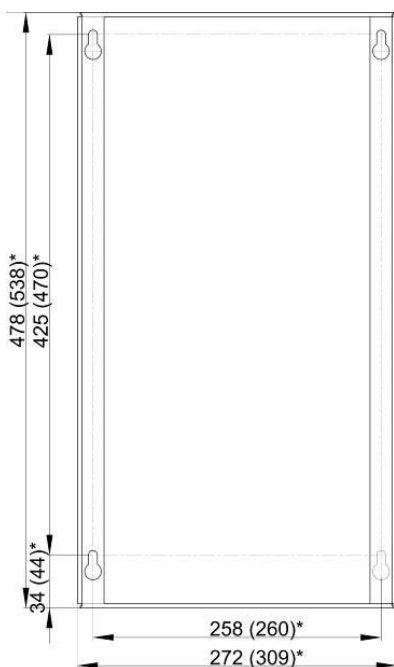
Рисунок 3. Крепление прибора на стену (размеры со звёздочкой* — для исполнения ST-20000, ST-30000)
