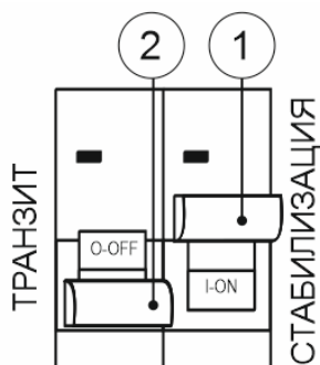
Переключатель типа «байпас»
