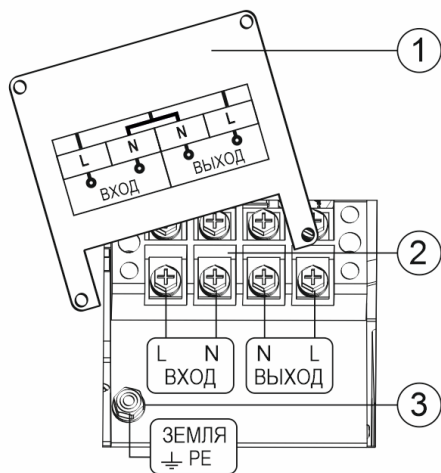
Рисунок 4. Схема подключения к клеммной колодке: 1. Съёмная крышка клеммной колодки; 2. Клеммная колодка; 3. Клемма заземления.
