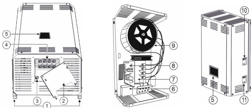
Рисунок 1. Общий вид стабилизатора и его функциональных блоков:
