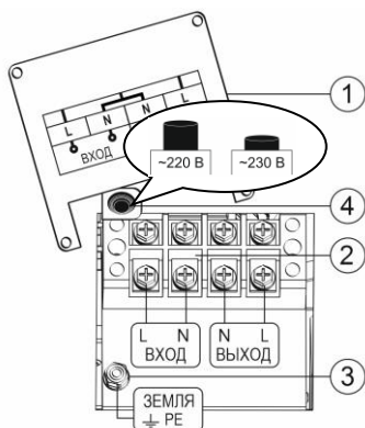
Рисунок 4. Схема подключения к клеммной колодке: 1. Съёмная крышка клеммной колодки; 2. Клеммная колодка; 3. Клемма заземления; 4. Кнопка переключения 220/230 В.
