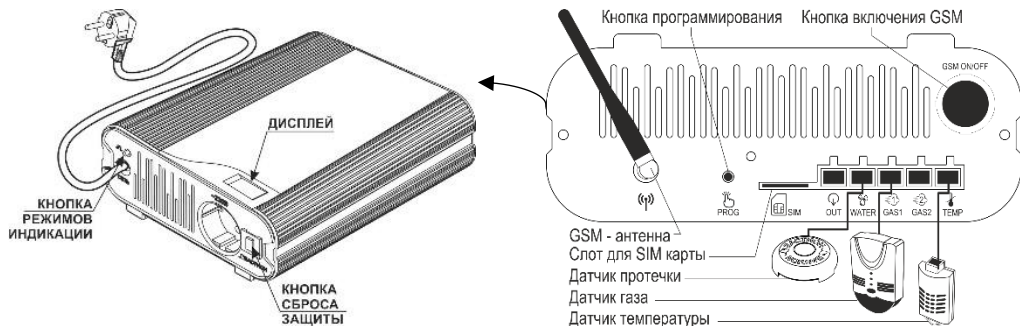
Рисунок 1- Общий вид системы
