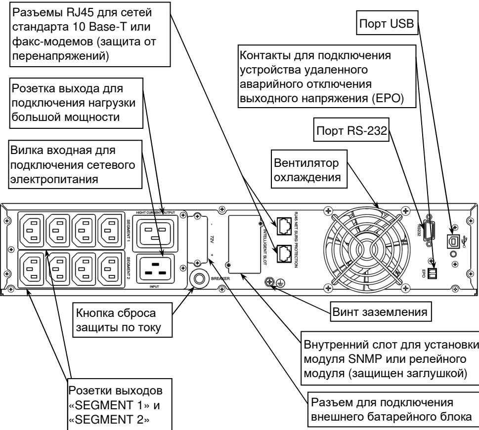
Рисунок 2 – Общий вид задней панели изделия.
