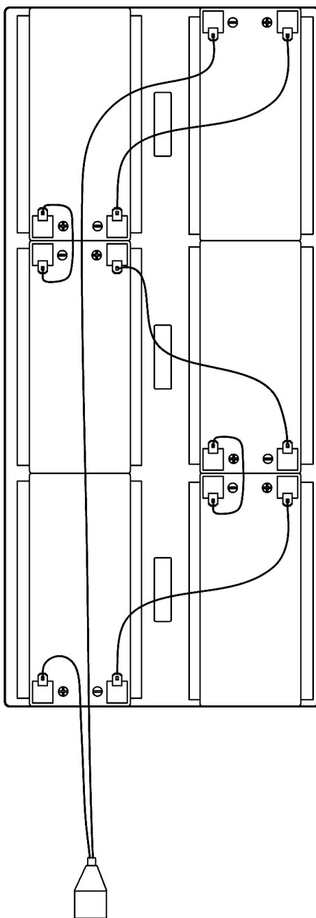
Рисунок 7 — схема соединений АКБ
