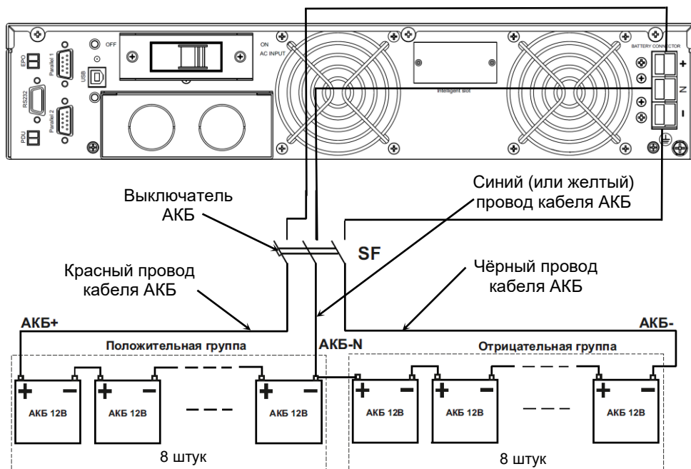
Рисунок 5 — Схема монтажа аккумуляторной батареи
