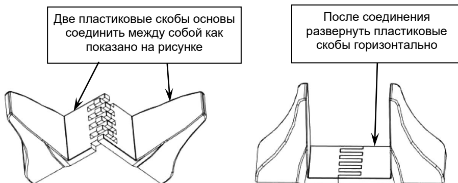
Рисунок 4 — Сборка пластиковых основ для вертикальной установки изделия
