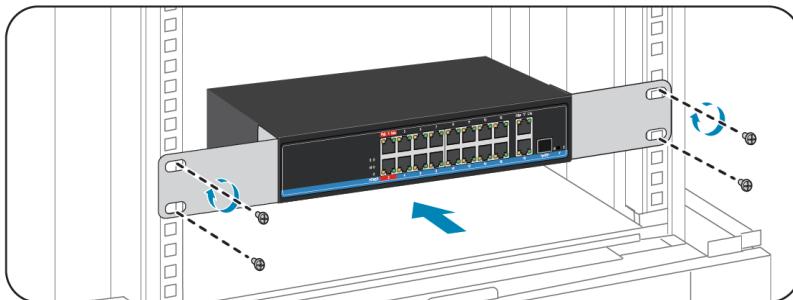
Рисунок 5 – крепление коммутатора на RACK-стойке
