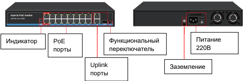
Рисунок 1 – передняя и задняя панель изделия
