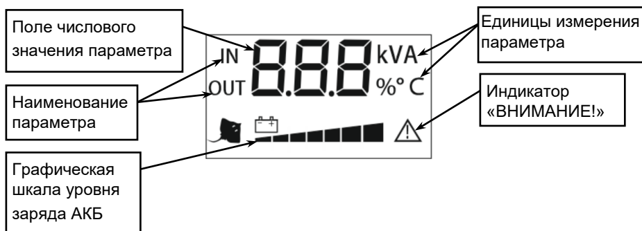
Рисунок 3 — Описание ЖК-дисплея
