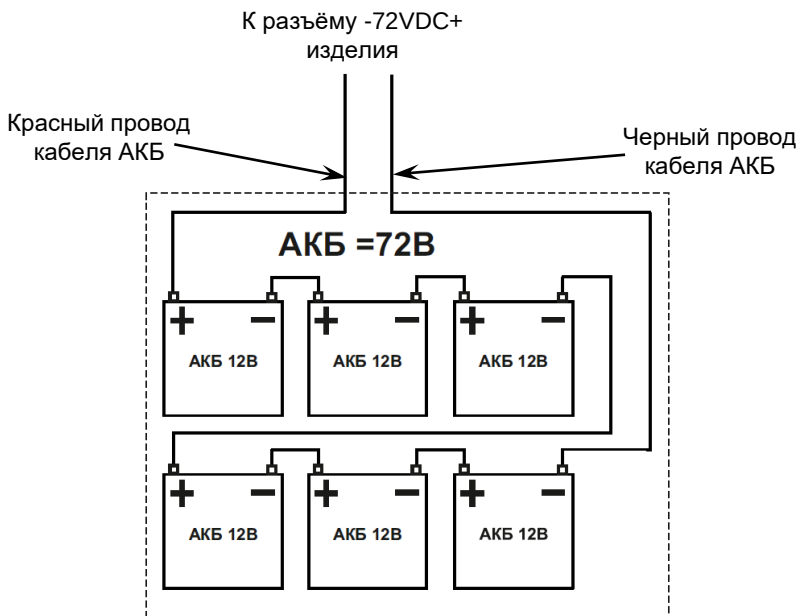
Рисунок 6 — Схема монтажа аккумуляторной батареи.
