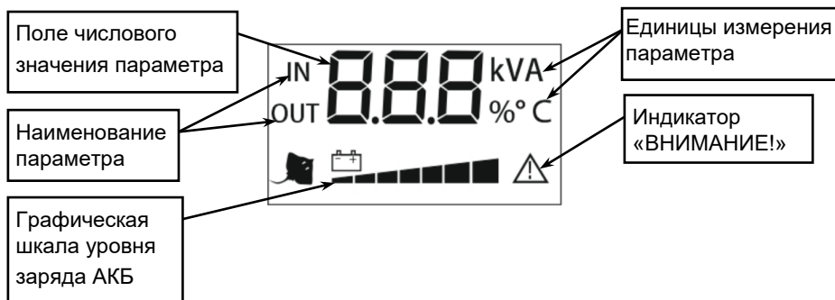
Рисунок 3 — Описание ЖК-дисплея
