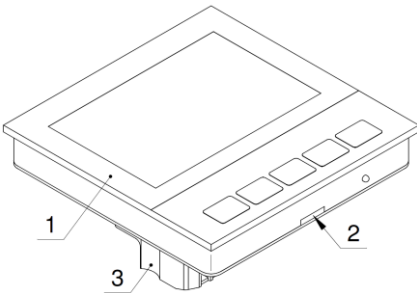
Рисунок 3 — Установка изделия
