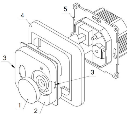
Рисунок 4 — Установка изделия.
