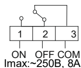
Рисунок 4 — Схема подключения нагрузки
