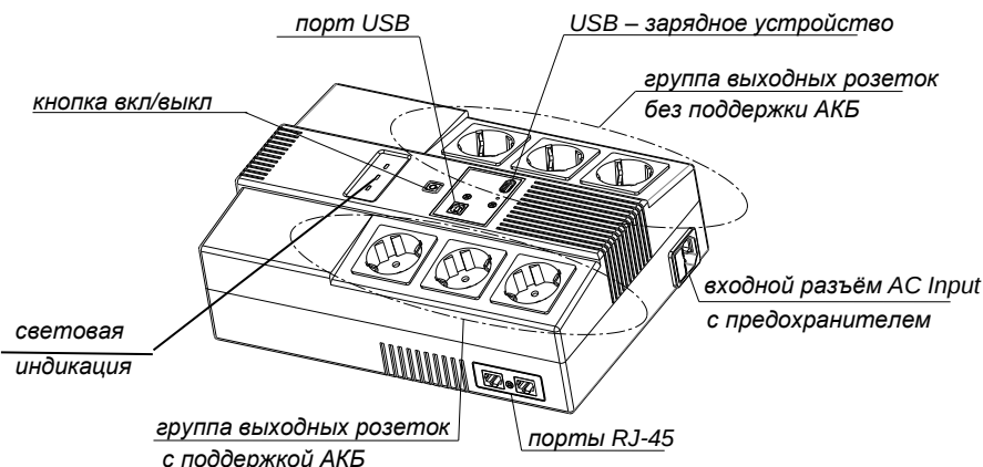
Рисунок 1 – Общий вид и элементы подключения
