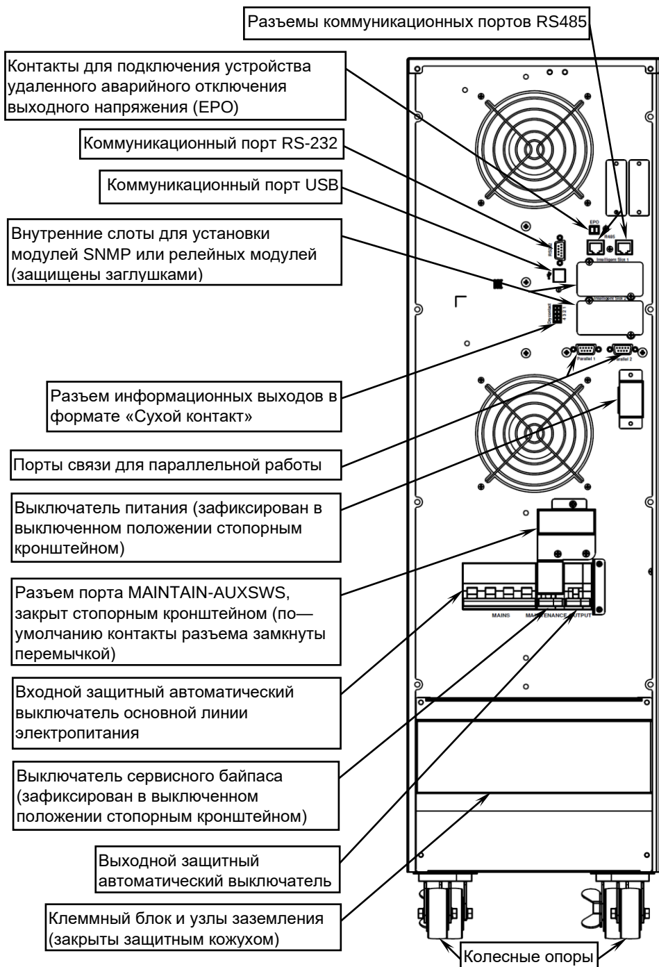
Рисунок 3 — Общий вид задней панели изделия
