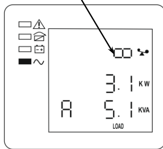
Рисунок 12 — ЖК-дисплей мощность нагрузки
