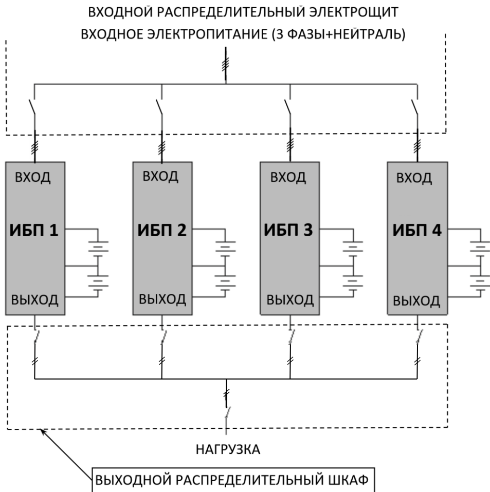
Рисунок 22 — Пример схемы подключения четырех изделий в систему параллельного резервирования с выходным распределительным шкафом.
