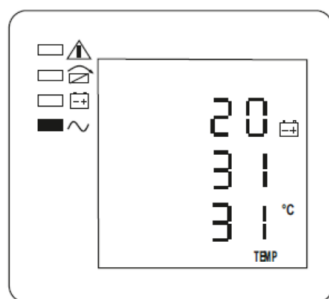
Рисунок 13 — ЖК-дисплей, температура АКБ, внутренняя и внешняя температура
