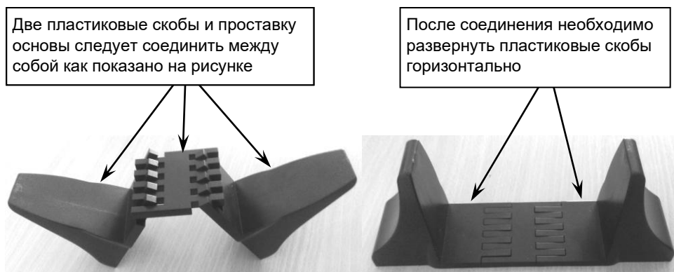
Рисунок 18 - Сборка пластиковых основ для вертикальной установки изделия.
