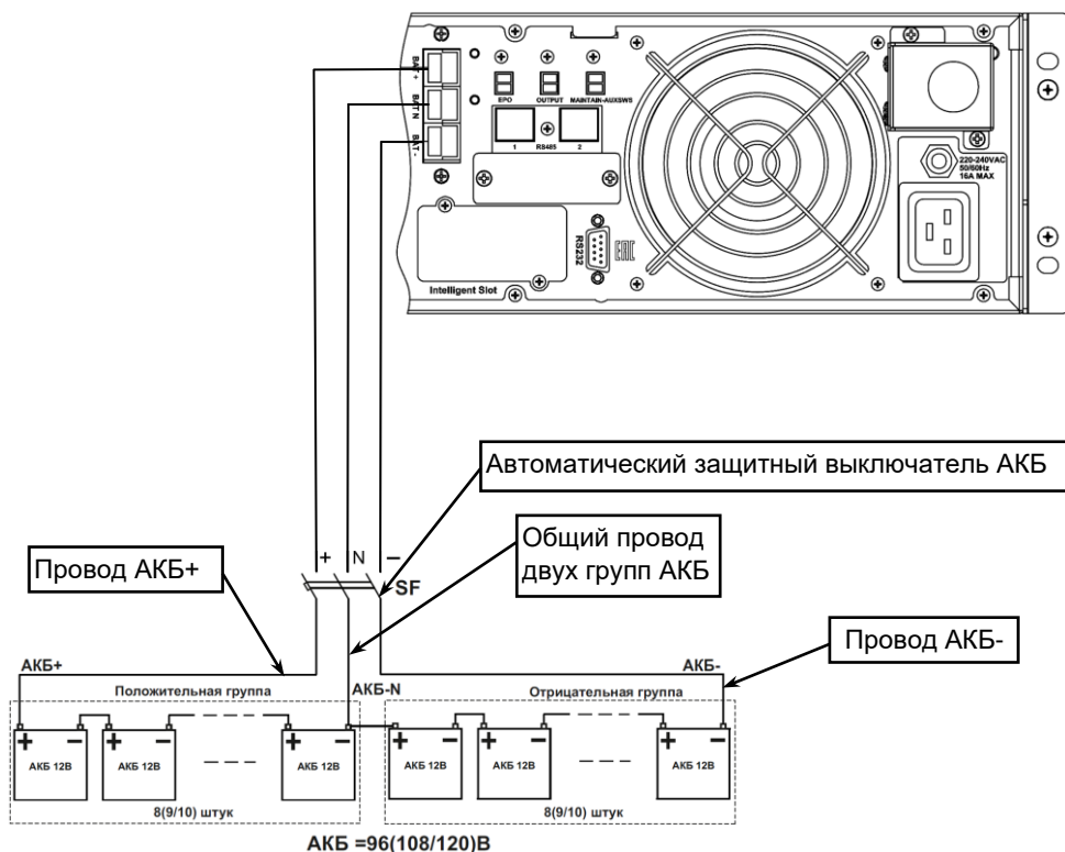
Рисунок 21 — Схема монтажа и подключения к ИБП аккумуляторной батареи.
