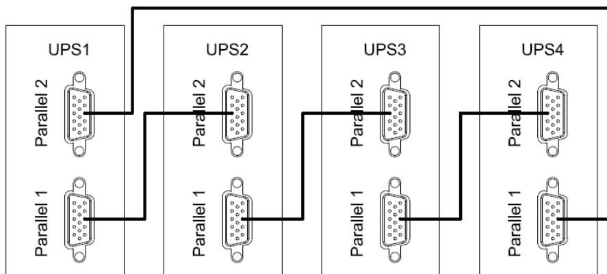
Рисунок 23 — Схема соединения изделий в «кольцо» через параллельные порты.
