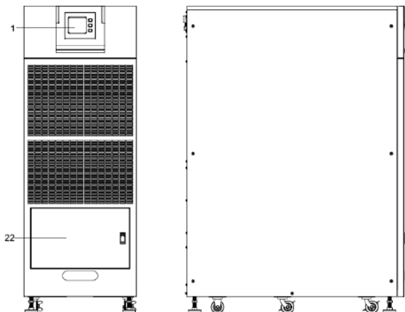
Рисунок 1 — Общий вид изделия спереди и слева
