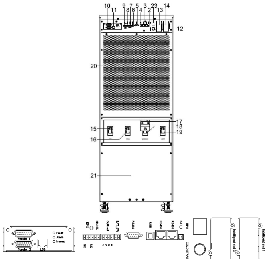
Рисунок 2 – Общий вид задней панели изделия
