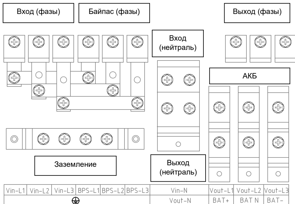
Рисунок 5 – Вид клеммных колодок изделия при трехфазном входе с питанием от одного источника, клеммы Vin и BPS соединены медными перемычками по трем фазам
