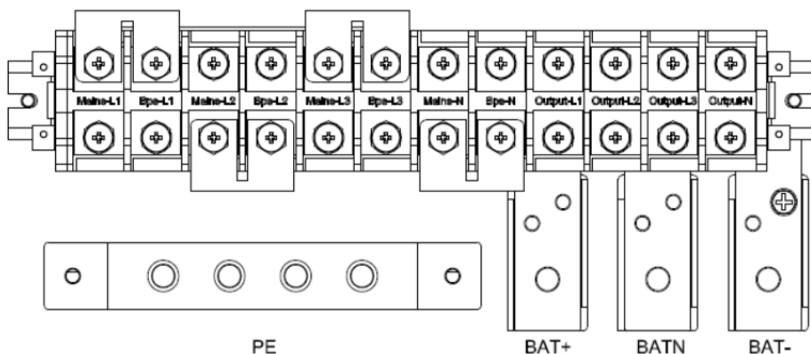
Рисунок 5 – Схема подключения изделия при одиночном входе для SKAT-UPS 80-3/3-ON, где клеммы Vin и BPS соединены медными перемычками по фазам и нейтралю
