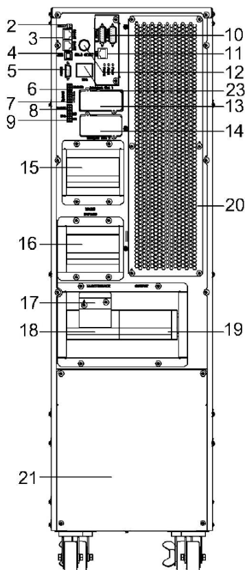
Рисунок 2 – Общий вид задней панели изделия
