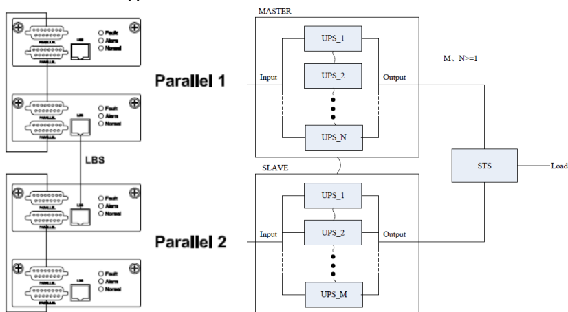
Рисунок 9 – Схема соединения изделий через LBS-кабель
