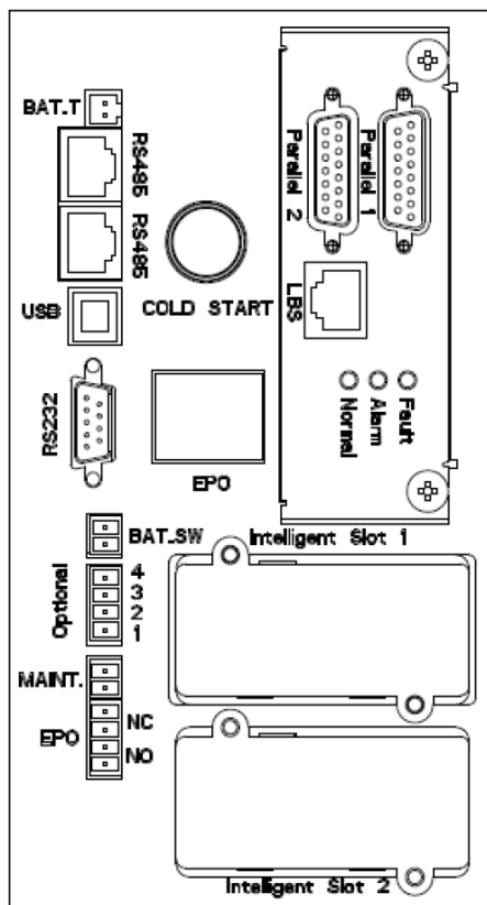
Рисунок 2 – Общий вид задней панели изделия, где
