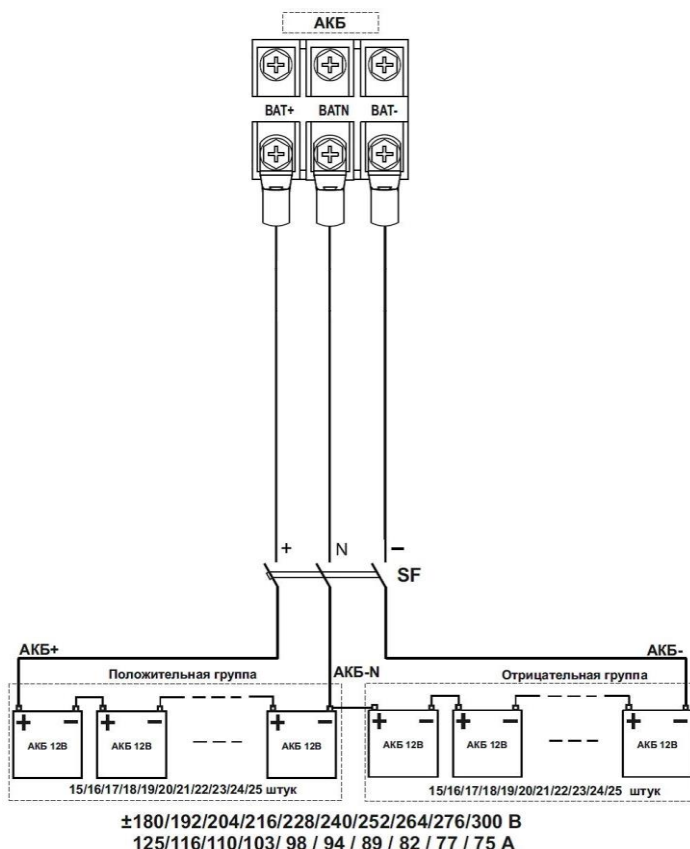
Рисунок 4 – Схема монтажа аккумуляторной батареи.
