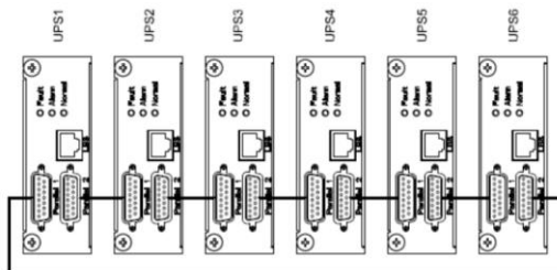
Рисунок 8 – Схема соединения изделий в «кольцо» через параллельные порты
