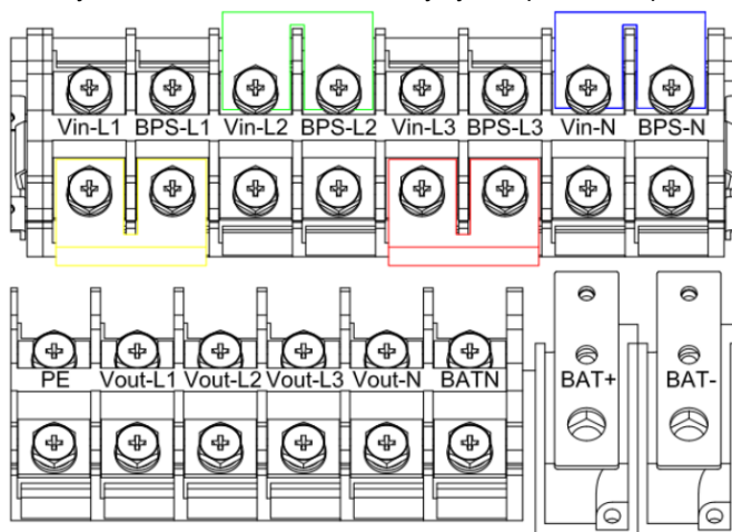
Рисунок 5 – Схема подключения изделия при одиночном входе, где клеммы Vin и BPS соединены медными перемычками по фазам и нейтрали
