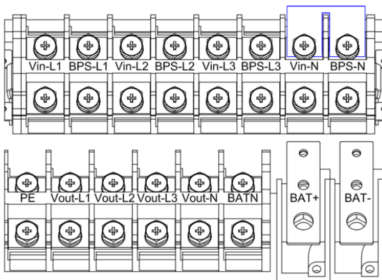
Рисунок 6 – Схема подключения изделия при двухканальном входе, где Vin-N и BPS-N соединены медной перемычкой
