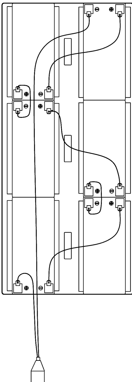
Рисунок 7 — схема соединений АКБ
