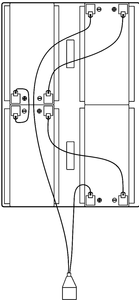
Рисунок 7 — схема соединений АКБ
