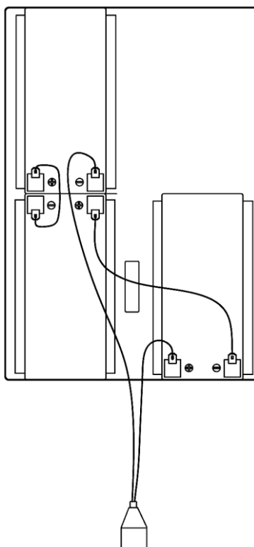
Рисунок 7 — схема соединений АКБ
