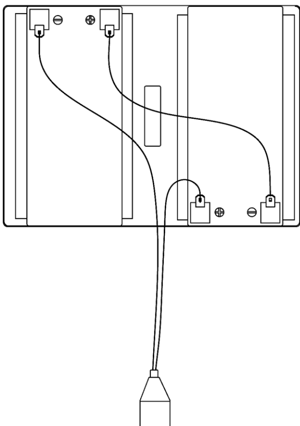
Рисунок 7 — схема соединений АКБ
