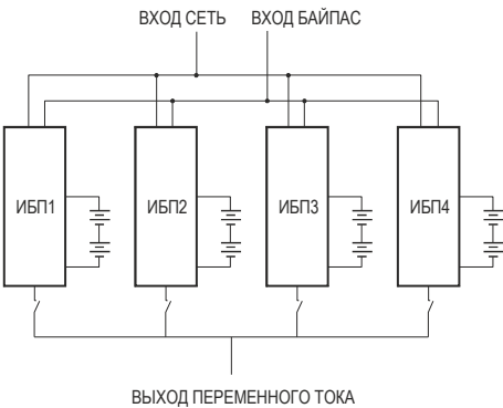
Рисунок 12 – Схема с разделным вводом байпас
