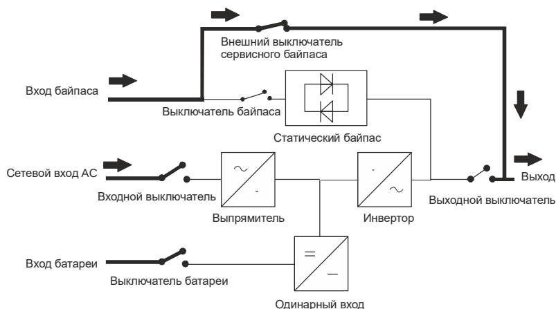
Рисунок 25 – Режим работы ручной байпас с раздельным вводом байпас
