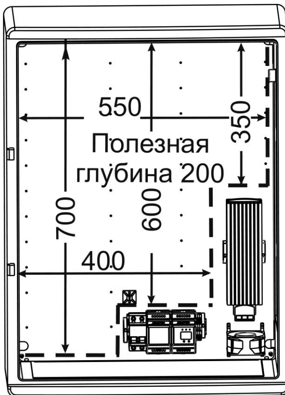
Рисунок 1 – Пространство внутри для установки доп. оборудования
