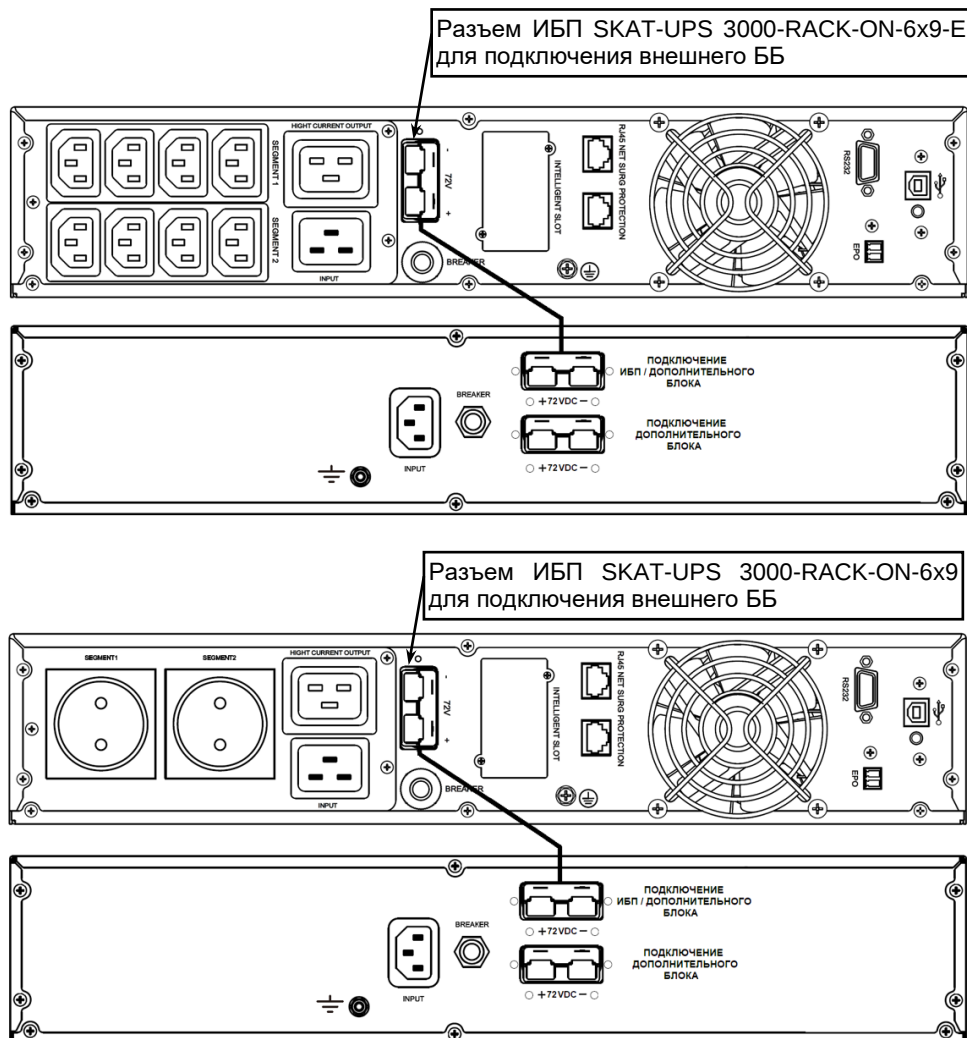
Рисунок 5 – Схемы подключения ББ к ИБП SKAT-UPS 3000-RACK-ON-6x9-E и SKAT-UPS 3000-RACK-ON-6x9
