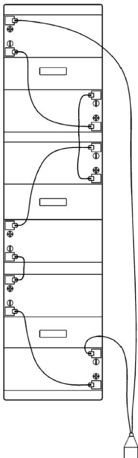
Рисунок 9 – Схема соединений АКБ в группе
