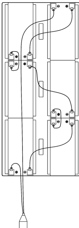
Рисунок 7 – Схема соединений АКБ
