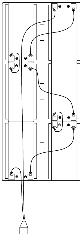
Рисунок 7 – Схема соединений АКБ
