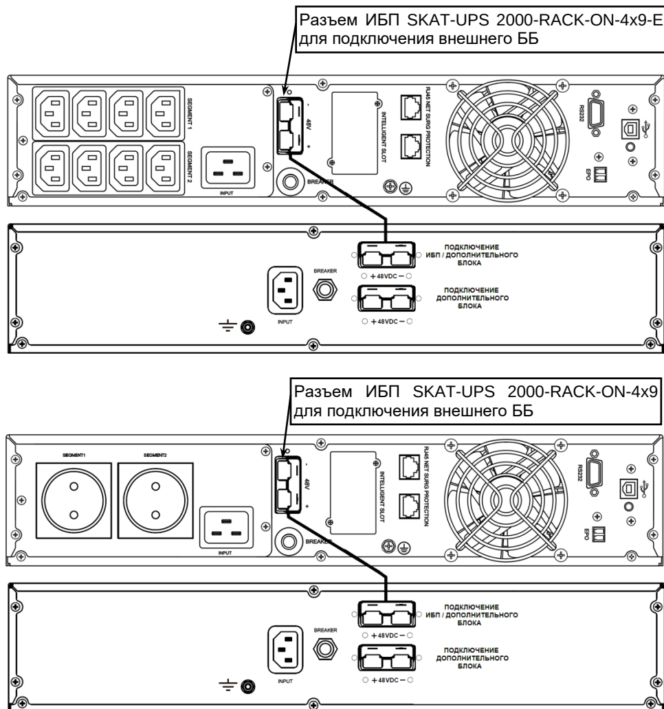
Рисунок 5 – Схемы подключения ББ к ИБП SKAT-UPS 2000-RACK-ON-4x9-E и SKAT-UPS 2000-RACK-ON-4x9
