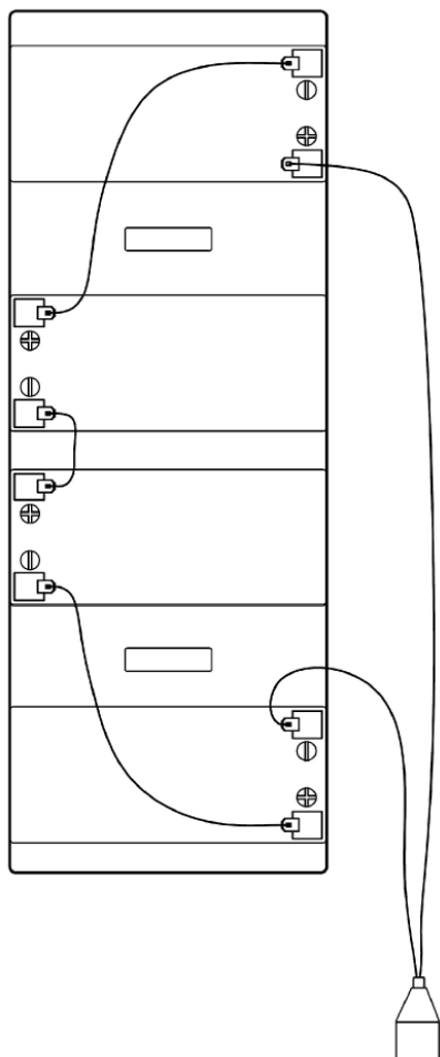
Рисунок 9 – Схема соединений АКБ в группе
