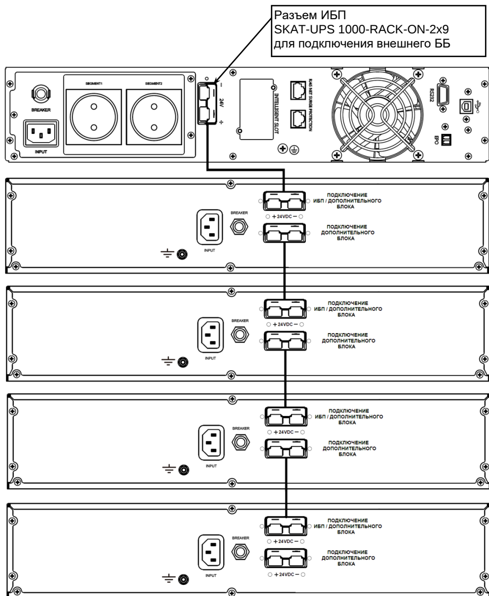
Рисунок 6 – Схема подключения нескольких ББ к ИБП (Начало на стр. 9)
