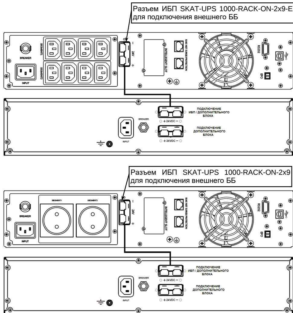
Рисунок 5 – Схемы подключения ББ к ИБП SKAT-UPS 1000-RACK-ON-2x9-E и SKAT-UPS 1000-RACK-ON-2x9
