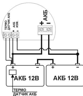
Рисунок 4 - Схема соединения аккумуляторов
