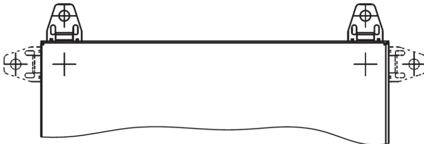
Рисунок 4 – пример установки кронштейнов
