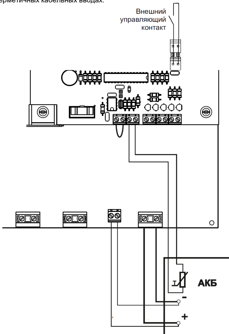
Рисунок 5 – Подключение АКБ, термодатчика и внешнего контакта
