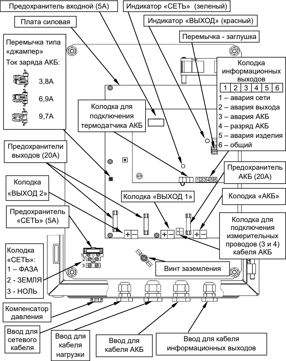
Рисунок 2 - вид изделия с открытой дверцей
