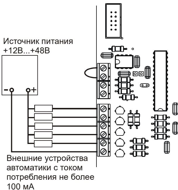
Рисунок 6 – Подключение внешних устройств автоматики.
