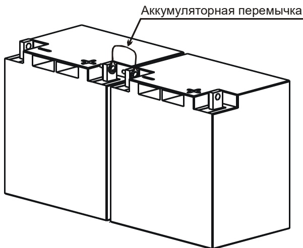
Рисунок 8 – схема последовательного соединения АКБ
