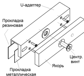
Рисунок 3 – Применение U-адаптера
