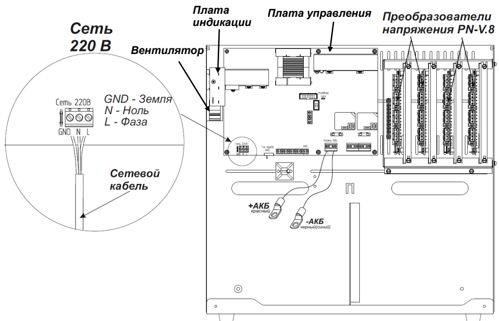
Рисунок 1 - Внешний вид изделия с открытой крышкой, подключение сетевых проводов и провода заземления
