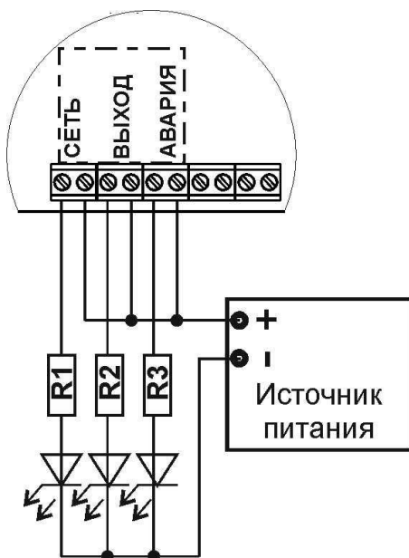
Рисунок 7– Подключение внешних индикаторов
