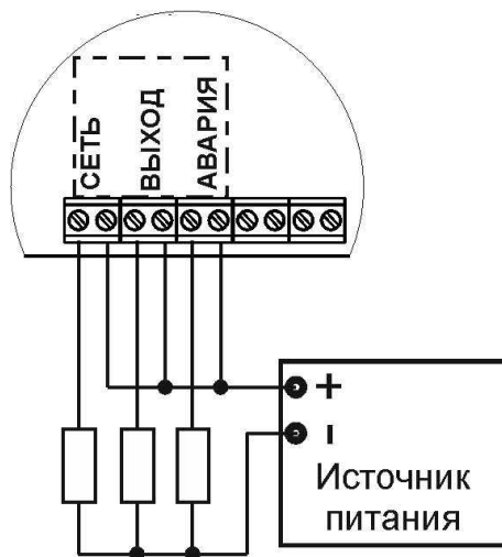
Рисунок 6 – Подключение внешних устройств автоматики
