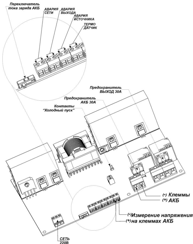
Рисунок 3 - Расположение органов коммутации, управления и защиты в зарядном устройстве
