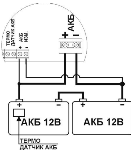
Рисунок 5 - Схема соединения аккумуляторов
