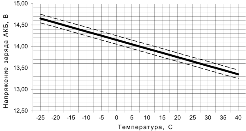
Рисунок 2 - Зависимость напряжения заряда АКБ от температуры
