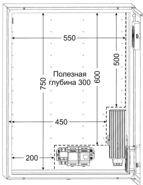
Рисунок 1 – Пространство внутри для установки доп. оборудования
