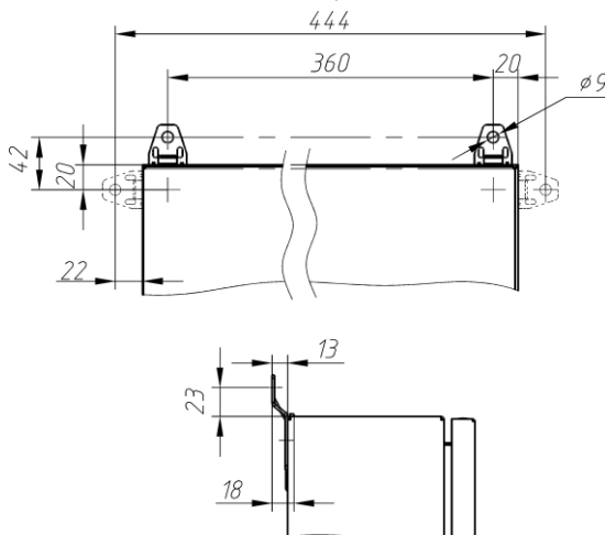
Рисунок 4 – Пример установки кронштейнов
