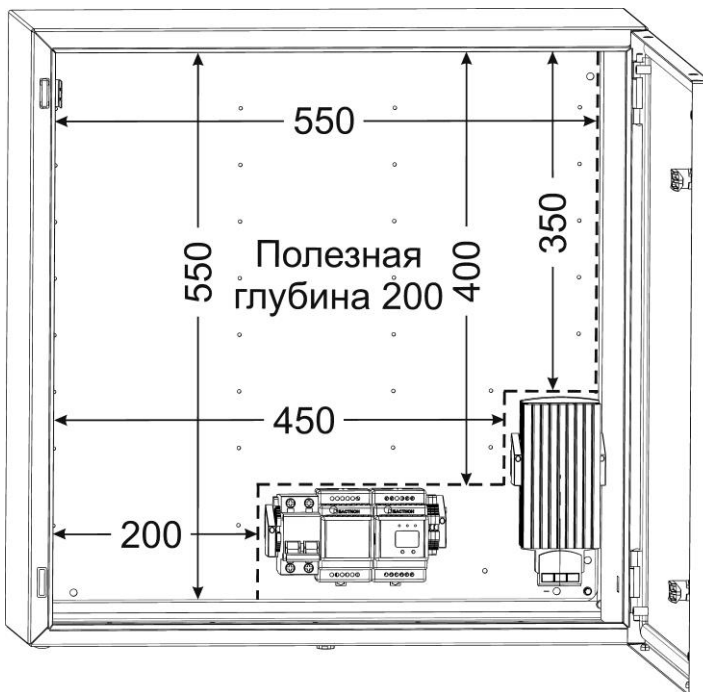
Рисунок 1 – Пространство внутри для установки доп. оборудования
