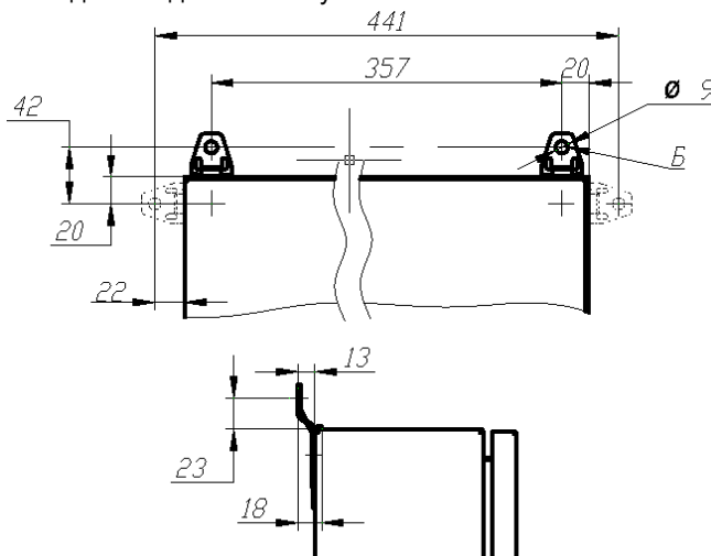
Рисунок 4 – Пример установки кронштейнов настенного крепления
