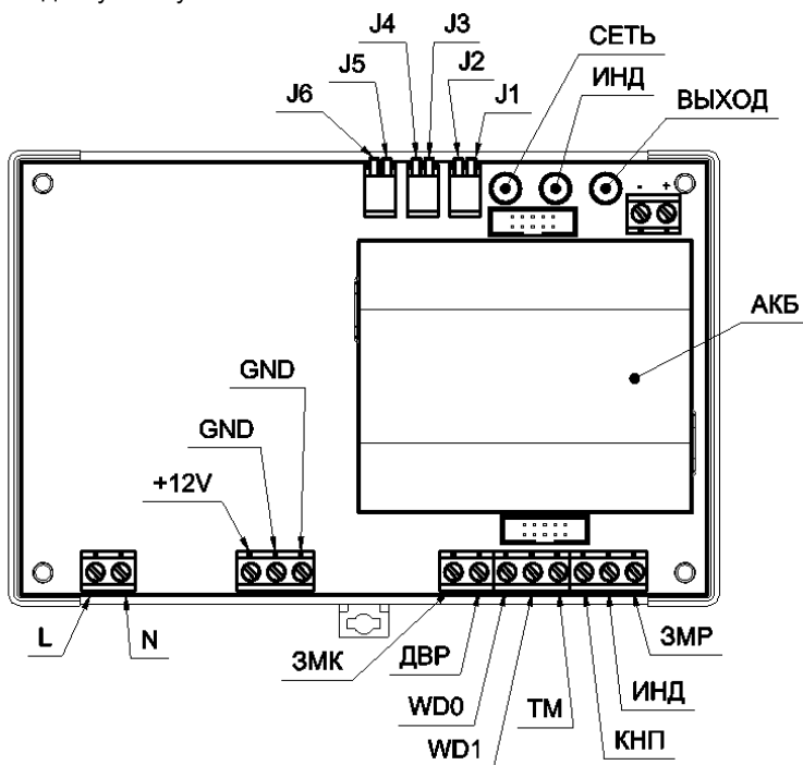
Рисунок 1 – Элементы подключения.
