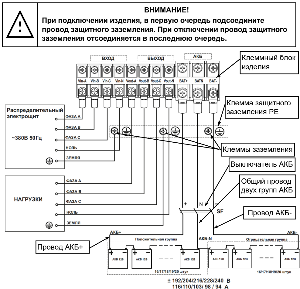
Рисунок 23 – Схема подключения изделия и монтажа аккумуляторной батареи.
