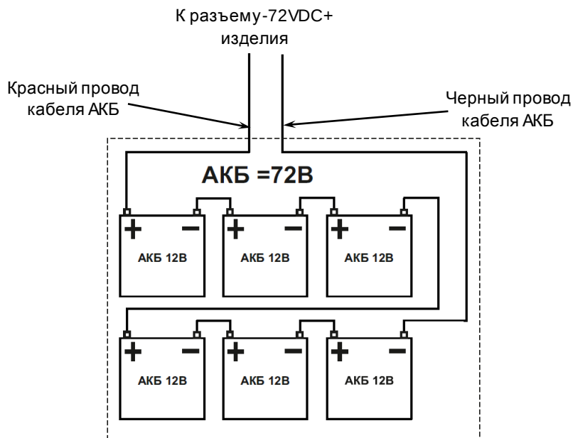
Рисунок 5 — Схема монтажа аккумуляторной батареи.
