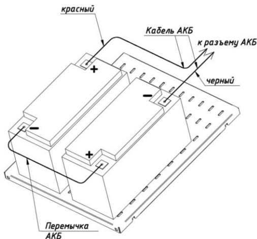
Рисунок 5 — Схема монтажа аккумуляторной батареи.
