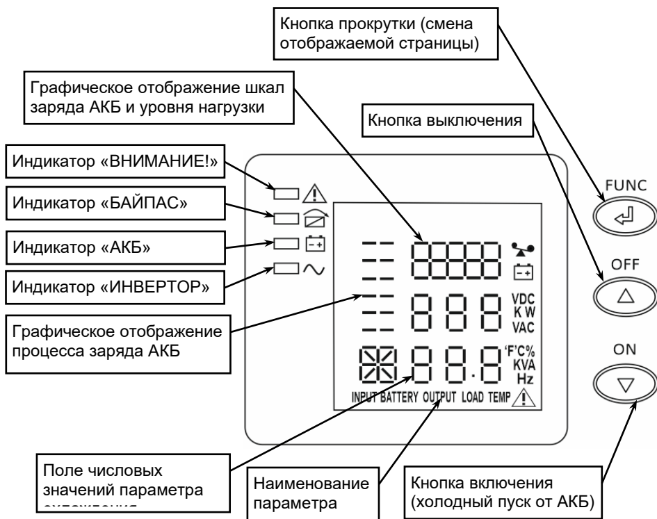
Рисунок 3 — ЖК—дисплей
