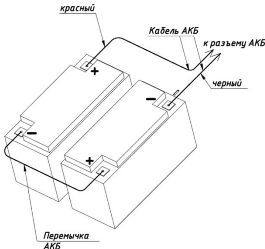
Рисунок 13 — Схема монтажа аккумуляторной батареи
