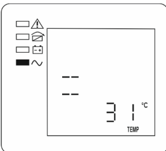
Рисунок 8 — ЖК-дисплей: отображается температура силовых узлов ИБП
