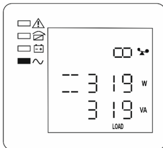
Рисунок 7 — ЖК-дисплей: мощность нагрузки на выходе, источник заряжает АКБ, напряжение на выход источника подается в режиме «ОСНОВНОЙ»
