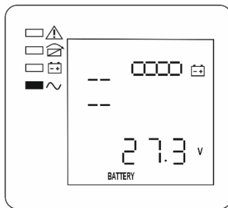
Рисунок 5 — ЖК-дисплей: напряжение на клеммах АКБ, степень заряда АКБ, источник заряжает АКБ, напряжение на выход источника подается в режиме «ОСНОВНОЙ»
