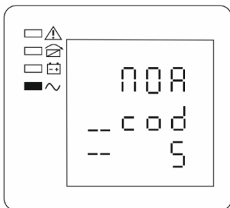
Рисунок 10 — ЖК-дисплей: режим работы и код состояния ИБП (см. таблицу 5)
