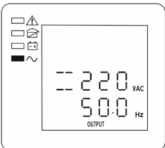
Рисунок 6 — ЖК-дисплей: выходные напряжение и частота, источник заряжает АКБ, напряжение на выход источника подается в режиме «ОСНОВНОЙ»
