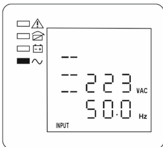
Рисунок 4 — ЖК-дисплей: входные напряжение и частота, источник заряжает АКБ, напряжение на выход источника подается в режиме «ОСНОВНОЙ»
