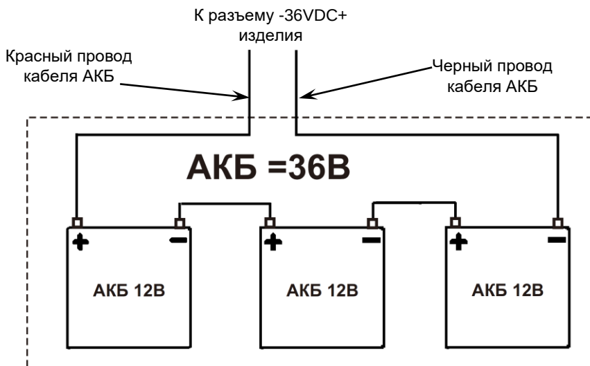
Рисунок 5 — Схема монтажа аккумуляторной батареи.
