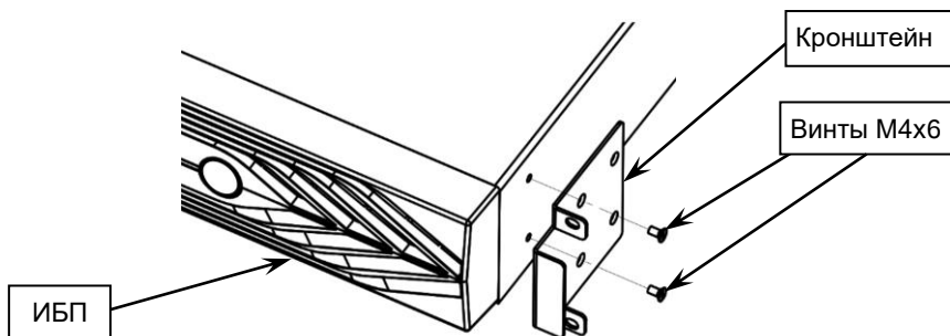
Рисунок 3 — Установка кронштейнов на корпус ИБП
