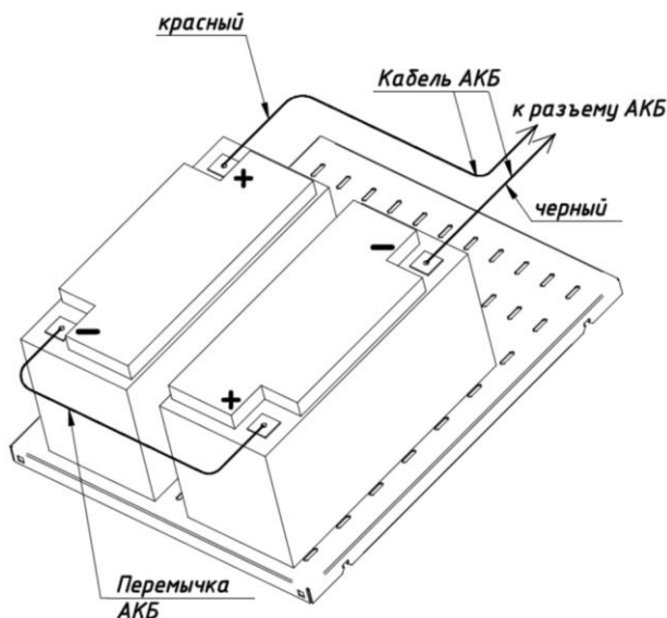
Рисунок 5 — Схема установки аккумуляторной батареи.
