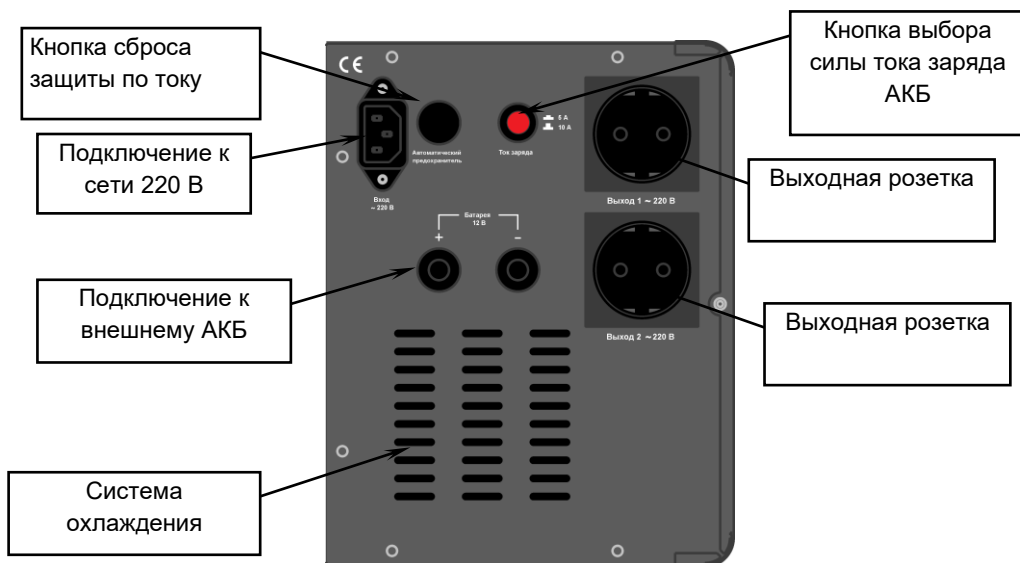
Рисунок 2.2 – Вид со стороны подключения изделий SKAT-UPS 333T, SKAT-UPS 555T
