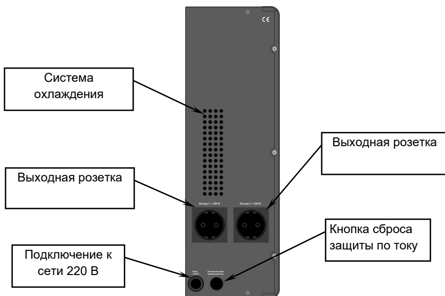
Рисунок 2.6 – Вид со стороны подключения изделий SKAT-UPS 2000T, SKAT-UPS 2500T
