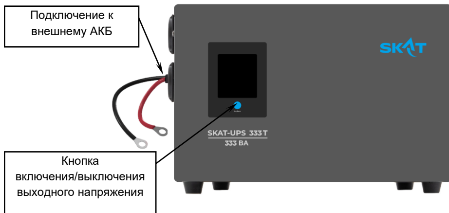
Рисунок 1.2 – Общий вид изделий SKAT-UPS 333T, SKAT-UPS 555T
