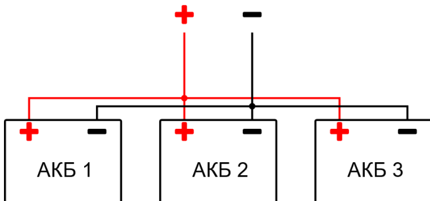
Рисунок 4 – Схема подключения АКБ
