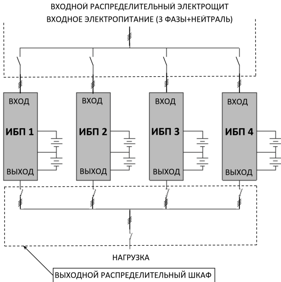
Рисунок 24 — Пример схемы подключения четырех изделий в систему параллельного резервирования с выходным распределительным шкафом.
