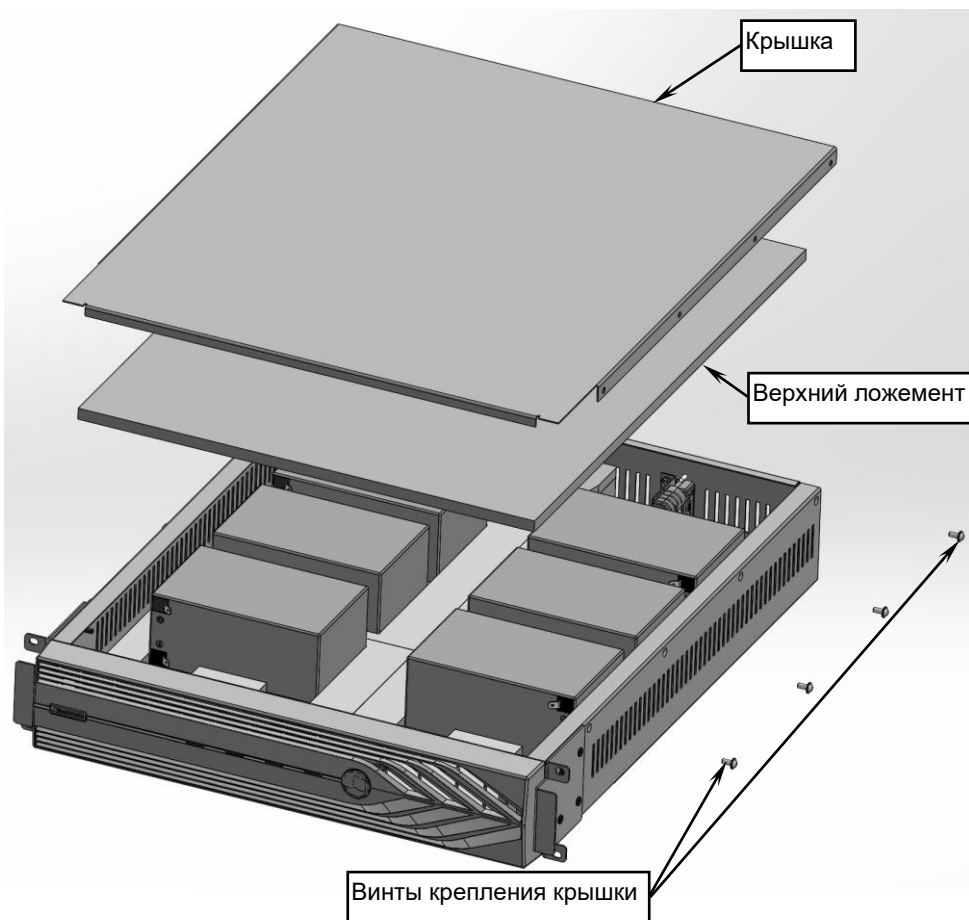
Рисунок 6 — Замена аккумуляторных батарей.
