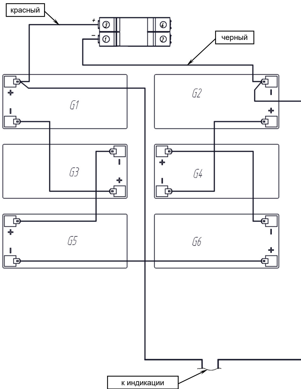
Рисунок 7 — Схема соединений аккумуляторных батарей
