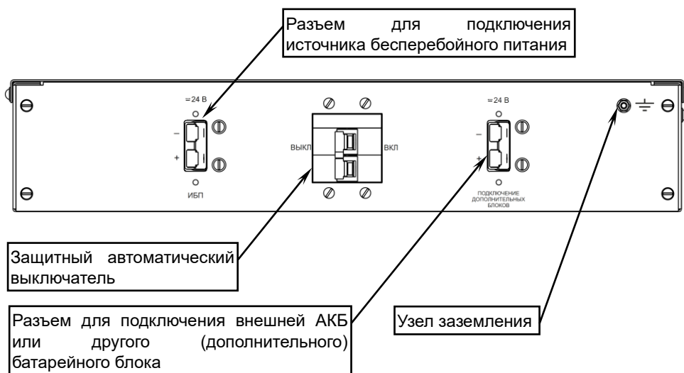
Рисунок 2 – Общий вид задней панели изделия со снятыми заглушками разъёмов
