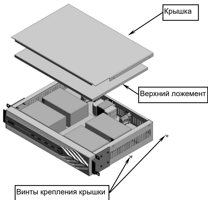
Рисунок 6 — Замена аккумуляторных батарей.
